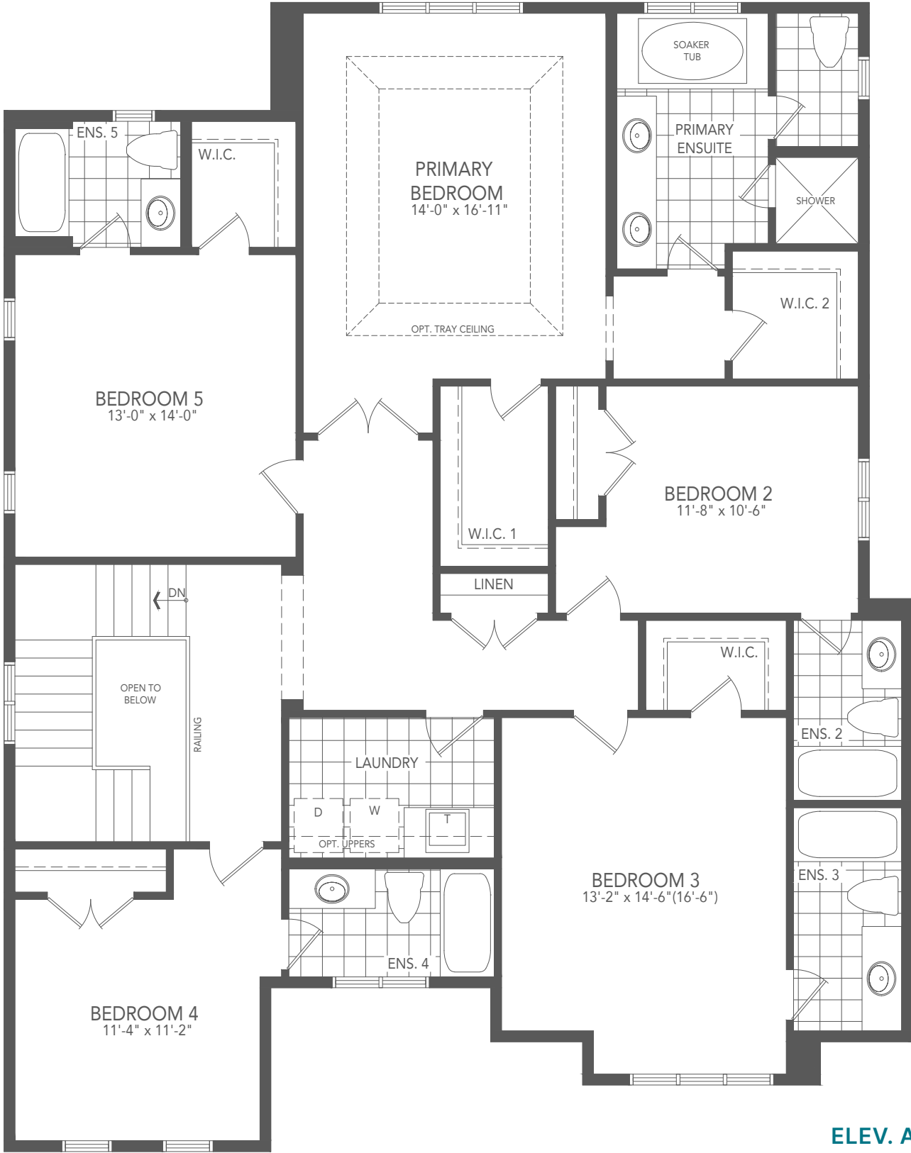
ELEV. A
