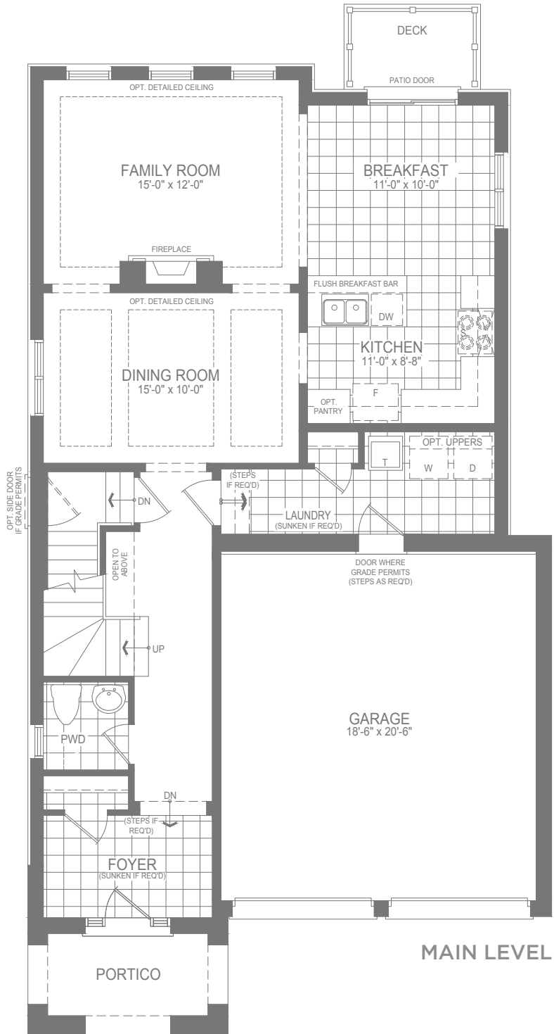
ELEV. C
