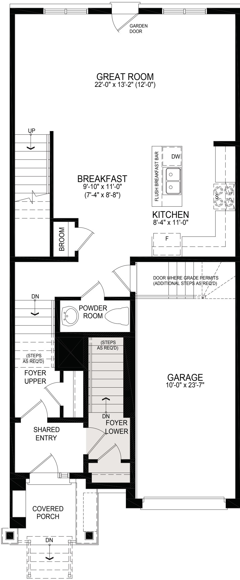
ELEV. B1
