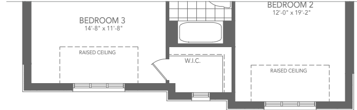
ELEV. C
