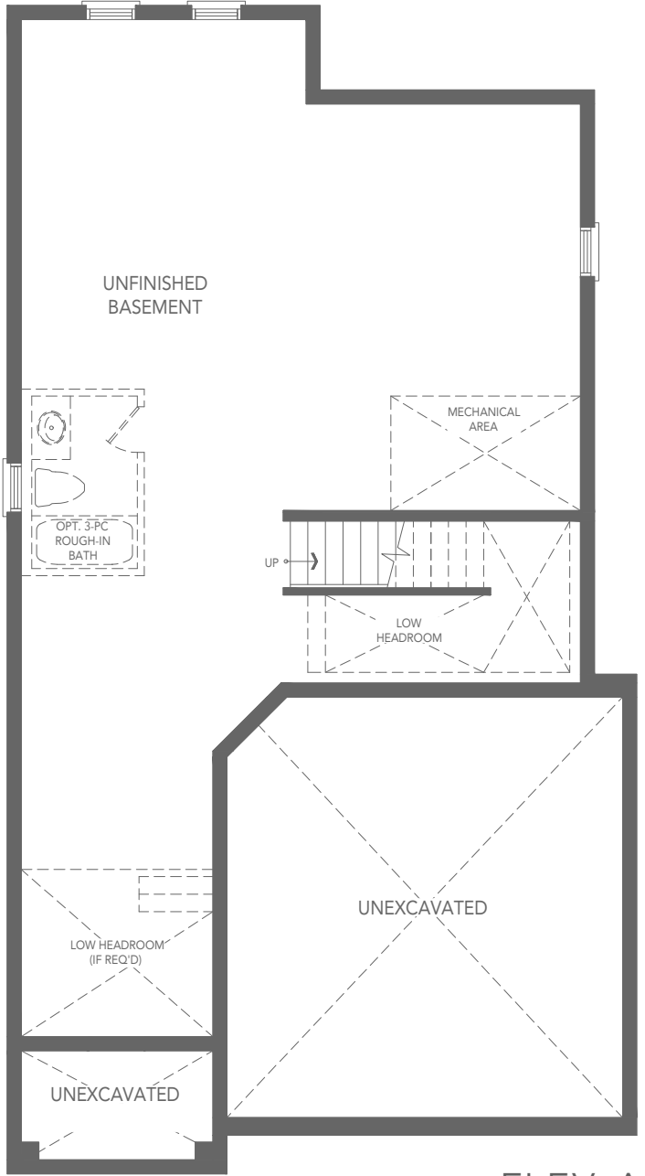
ELEV. A
