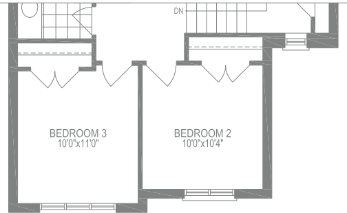
ELEV. D
