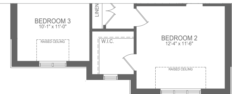
ELEV. C
