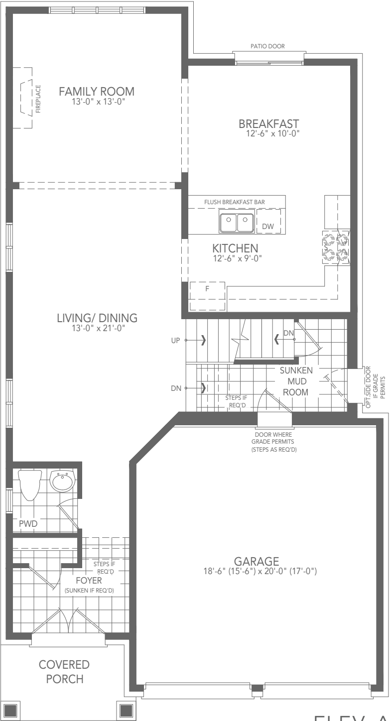
ELEV. A
