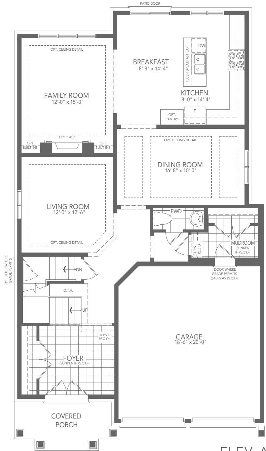
ELEV. A
