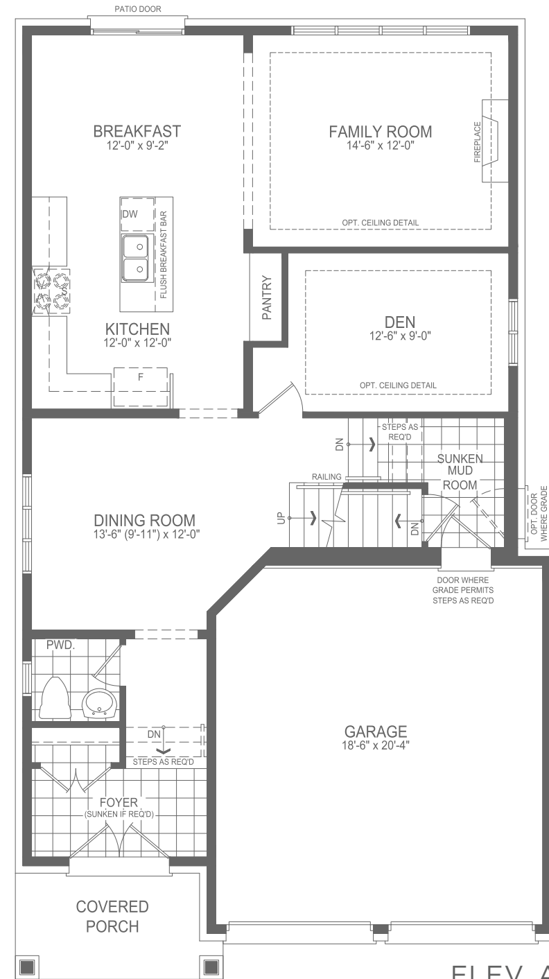
ELEV. A
