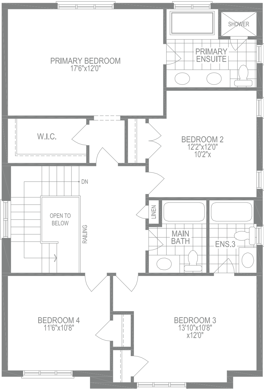
ELEV. A
