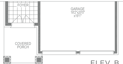
ELEV. B
