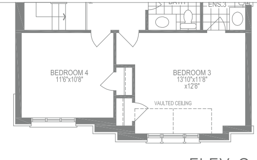
ELEV. C
